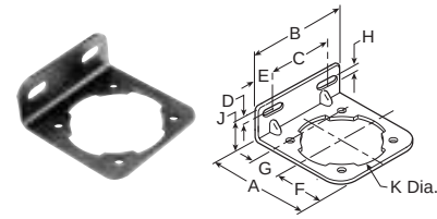
L-Bracket GPA-96-605
