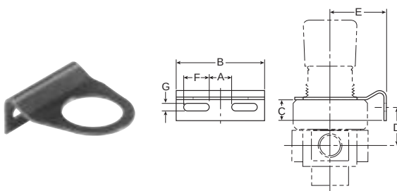
L-Bracket GPA-96-313
