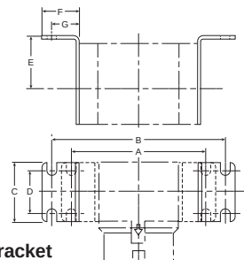
L-Bracket P3NKA00MW
