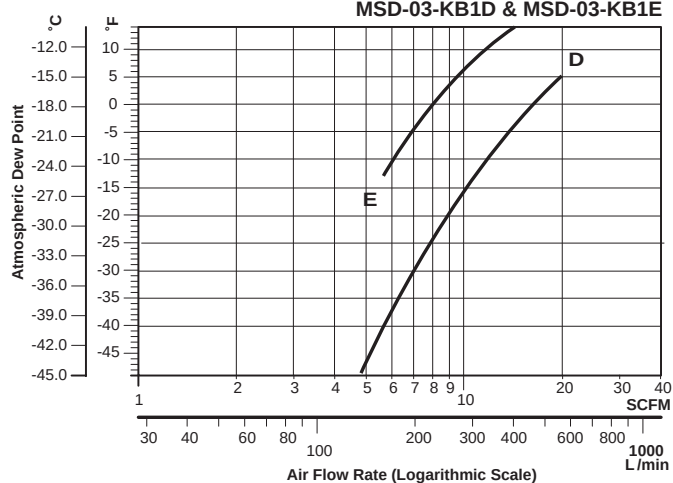
MSD-03-KB1D &amp; MSD-03-KB1E
