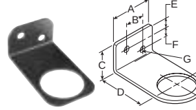
L-Bracket GRP-95-147
