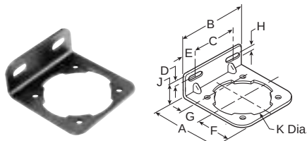
L-Bracket GPA-96-605
