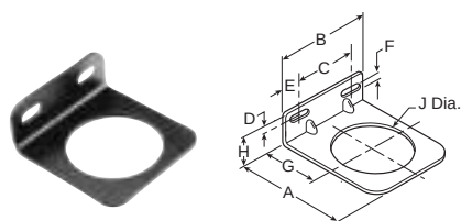
L-Bracket GRP-96-606
