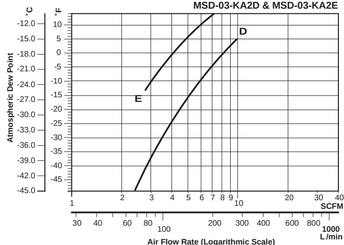
MSD-03-KA2D &amp; MSD-03-KA2E
