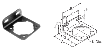
L-Bracket GPA-96-604
