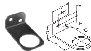
L-Bracket GRP-95-147
