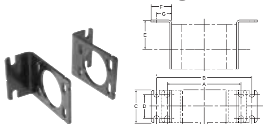
L-Bracket P3NKA00MW
