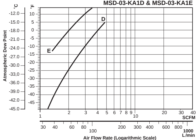
MSD-03-KA1D &amp; MSD-03-KA1E
