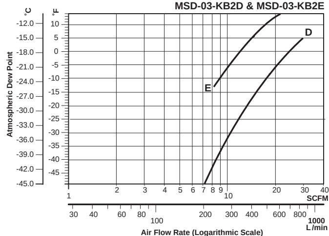
MSD-03-KB2D &amp; MSD-03-KB2E
