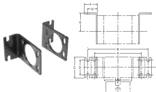
L-Bracket P3NKA00MW
